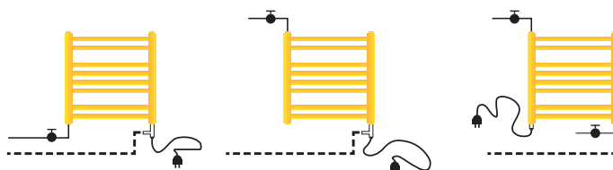
Примеры схем подключения электрического нагревательного элемента GRZ к радиатору
