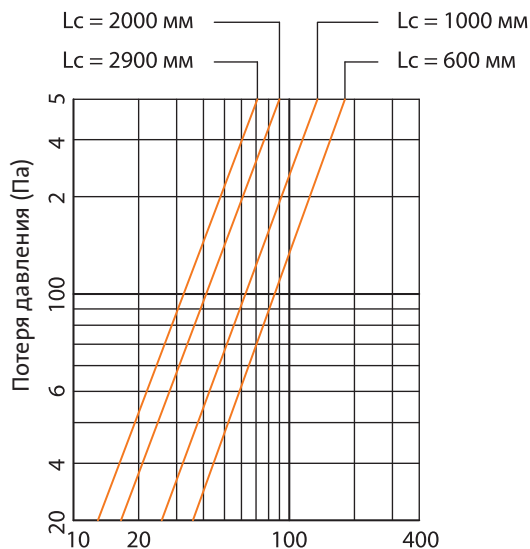
Массовый расход воды (кг/ч)
